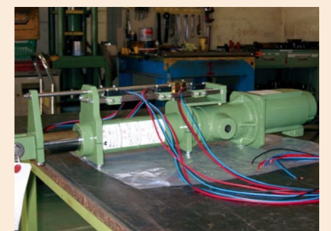
AC100Vモータ 推力:196N 小型防水シリンダ 輪受洗浄装置用
