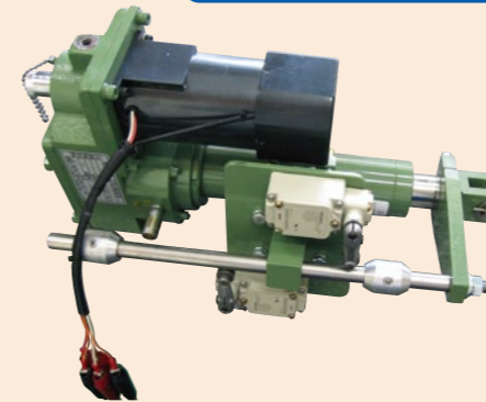
AC100Vモータ 推力:4.9KN 小型シリンダ
